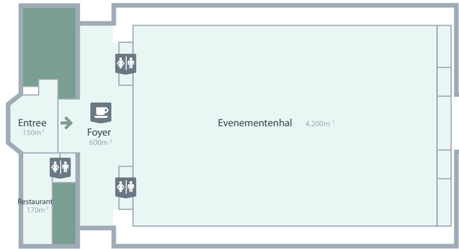
Begane grond
